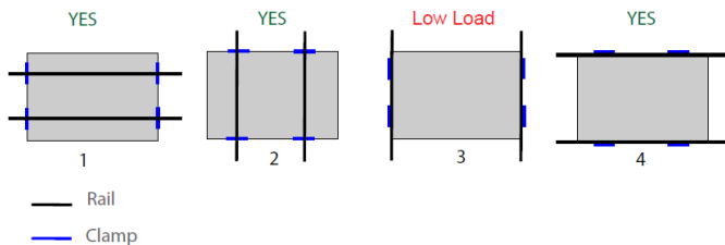
図 3. 架台の構成
