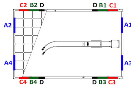
Figure 2 : Position des brides ou attaches de fixation pour les panneaux Maxeon
