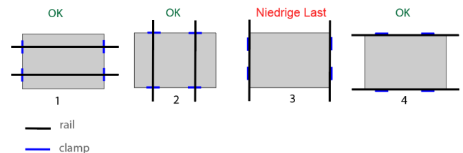
Abbildung 3: Montagekonfigurationen
