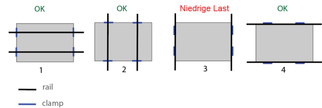
Abbildung 3: Montagekonfigurationen
