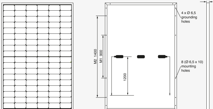
Abb. Prinzipskizze
